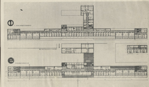
Grundrisse des Erd- und ersten Obergeschosses
