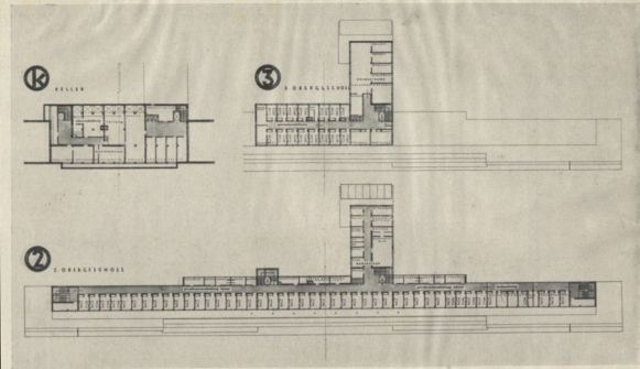
2 Grundrisse des 2. und 3. Obergeschosses und des Keller
